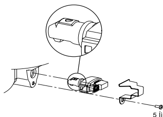
Рис. 45 Правильное положение датчика
