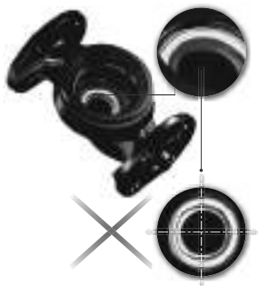
Рис. 16 Неправильно выровненная система уплотнений
