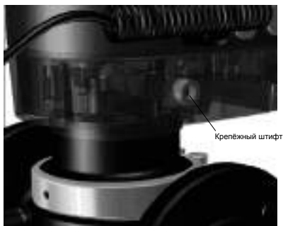
Рис. 12 Крепежный штифт для модификаций с подключением через штекер
